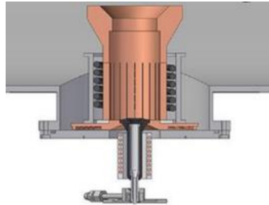
Close-up of pour tube and gas nozzle
