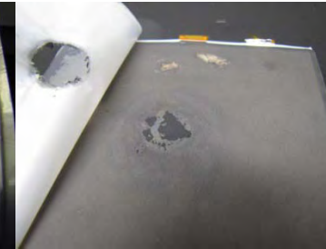
Anode electrode
