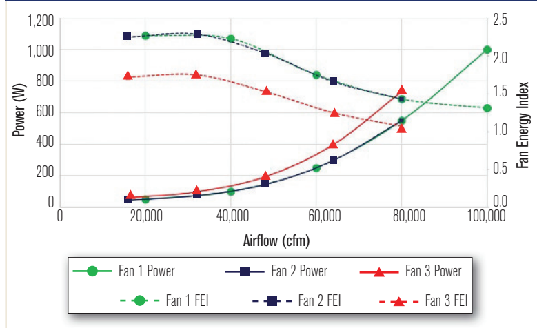
FIGURE 2 Fan performance data for Fan 1, Fan 2 and Fan 3 from Table 2 .
