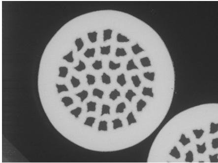
Rotor Strand:
