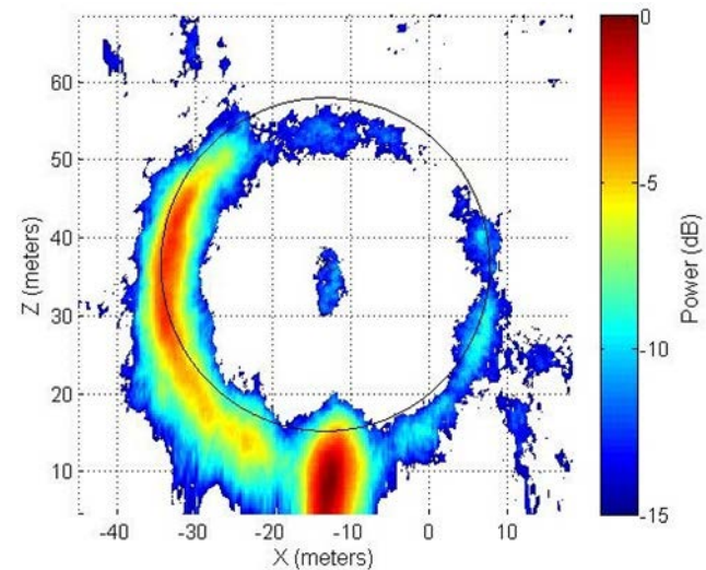
Yaw error = 31°
