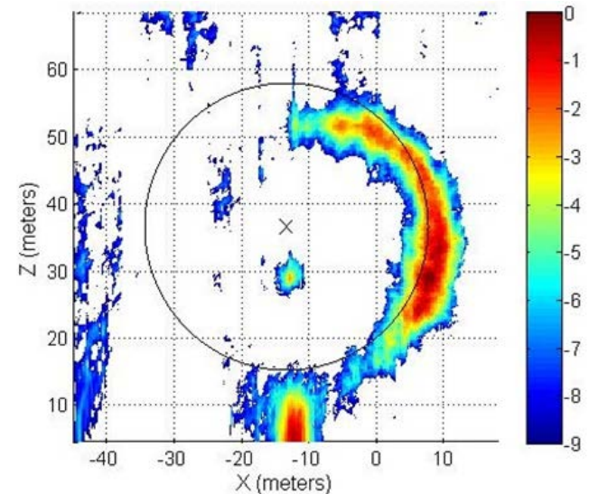
Yaw error = 2°
